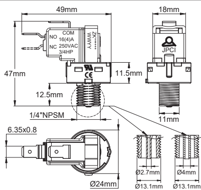
Rosca 1/4 NPSM
